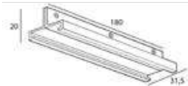
MHT1-P2-WH UCHWYT DO SZYN, DŁUGI, BIAŁY track bracket, long, white
